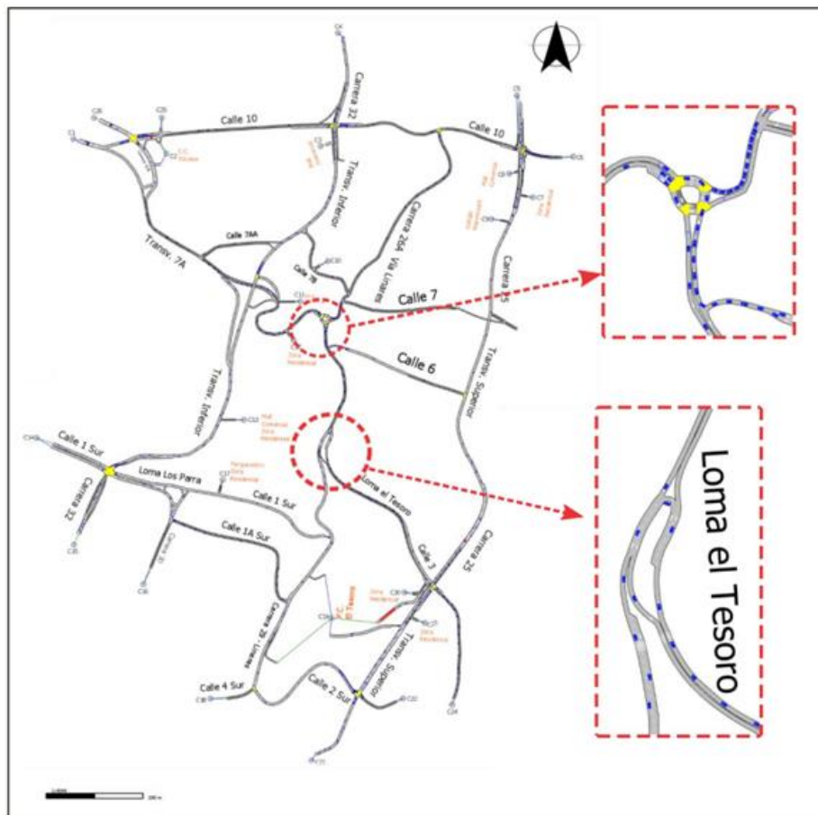
Figura 46 . Comportamiento del flujo vehicular – Escenario 8
